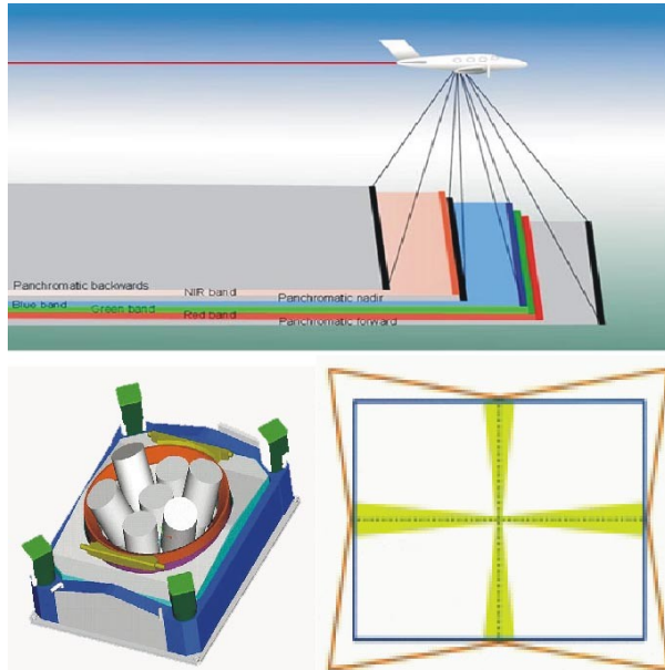
Abb.2: Die neuen digitale Luftbildkameras der beiden führenden Photogrammetrie-Hersteller. Während Leica (oben) einen multispektralen Zeilenabtaster verwendet, setzt Z/I auf ein Bündel von Kameras mit flächigen (2D-) Sensoren: Links unten das Schema des Kamerablocks, rechts die Zusammensetzung des Bildmosaiks aus 4 Einzelbildern)
