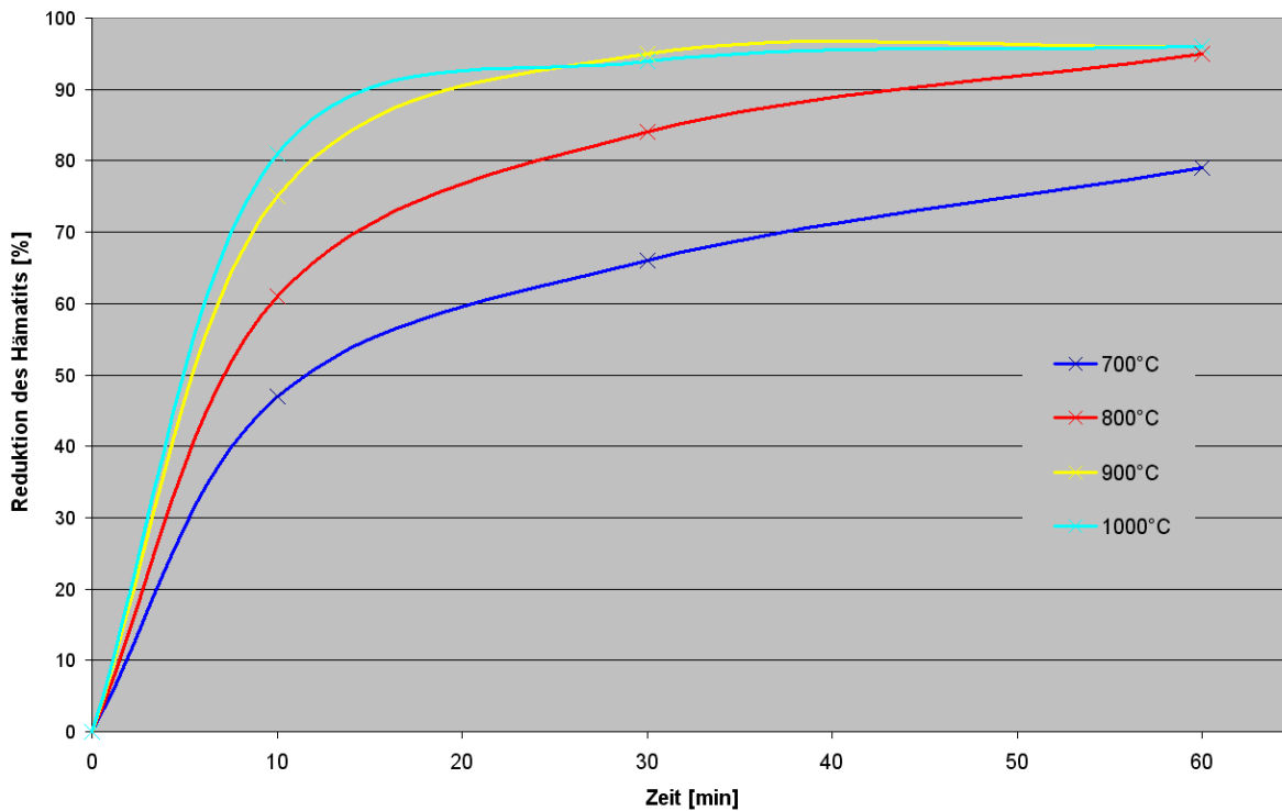
Bild 4.56 Reduktion des Hämatits mit Kohlenmonoxidgas
