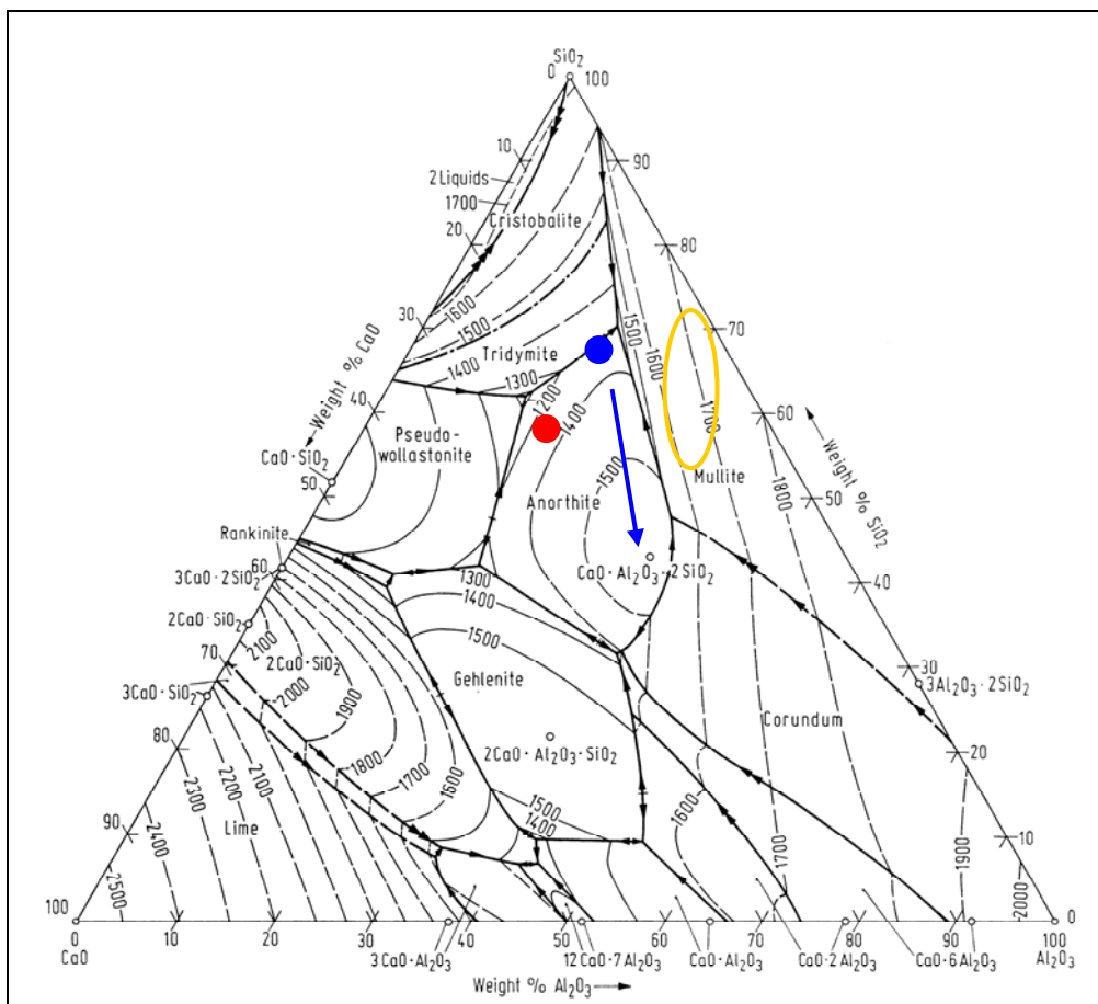
Bild 4.39 Dreistoffsystem Calciumoxid-Aluminiumoxid-Siliciumoxid
