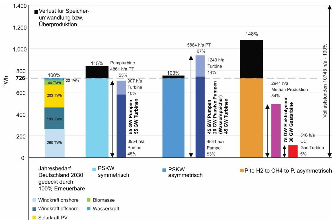
Abb. 4. Speichervergleich, Basisjahr 2019, extrapoliert für 100% erneuerbaren Strom in Deutschland für 2030, PSKW symmetrisch (Pumpleistung = Turbinenleistung), PSKW asymmetrisch (mit passiver Speicherung in großen Speicherseen), Speicherung über Wasserstoff und Rückverstromung über Gaskraftwerke
