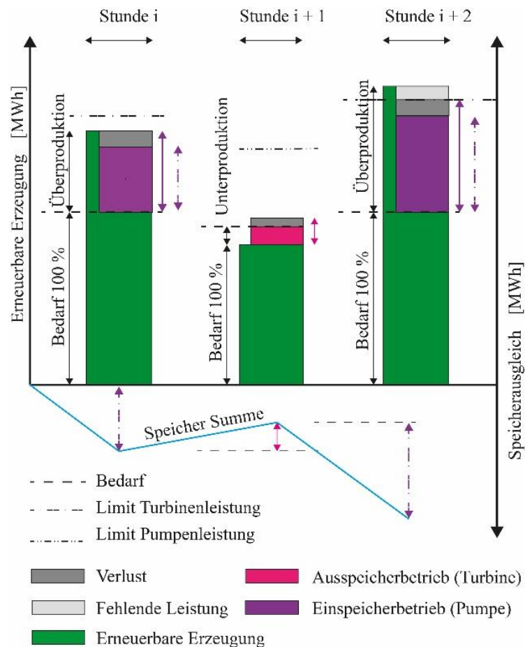
Abb. 1. Methodik der Speicherbilanz auf stündlicher Erzeugungsbasis
