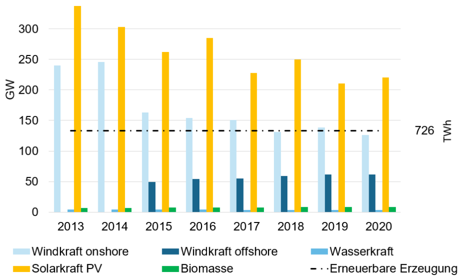
Abb. 2. Extrapolierter erneuerbaren Installation je Basisjahr um den Bedarf 2030 zu decken
