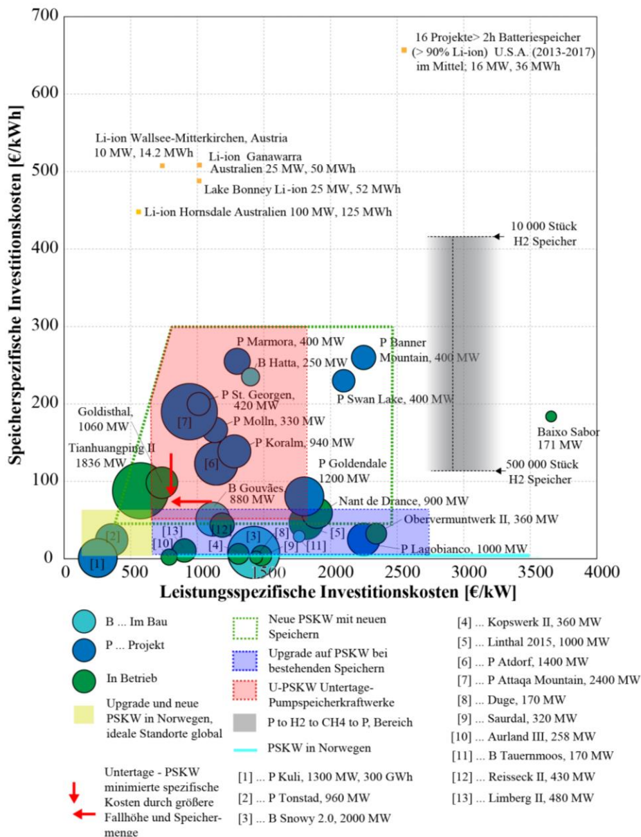
Abb. 5. Spezifischer Kostenbereich für Kapazität € / kW und Energie € / kWh für Speichersysteme, verschiedene PSKW-Projekte, Technologiebereich von PSKW und U-PSKW, Li-Ionen-Batterieprojekte (Richter, 2020) (Pikl, Richter, & Zenz, 2019) (Saha, 2020) (Pitorac, Vereide, & Lia, 2020) mit Kostenbereich, Kostenbereich von Leistung zu H2 bis CH4 zu Leistung (PtGtP) Anlagen (van Leeuwen & Zauner, 2018) (Theodoropoulos, Daly, & Dinan) (James, Houchins, Huya-Kouadio, & DeSantis, 2016), (initiale Grafikdaten und Layout basierend auf (Pikl, Richter, & Zenz, 2019))
